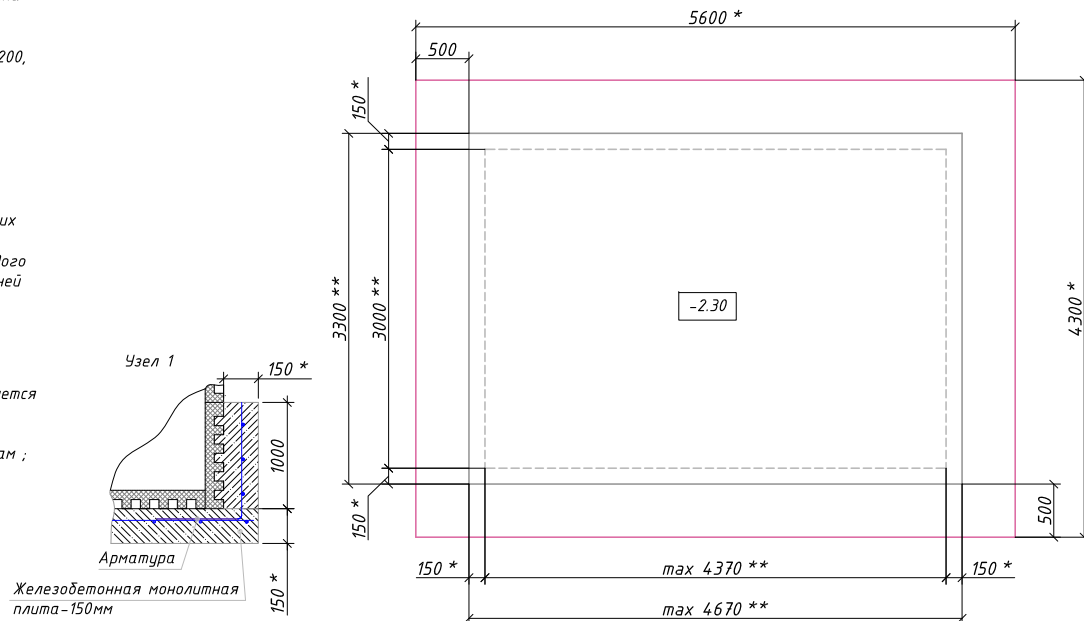
План котлована с плитой
