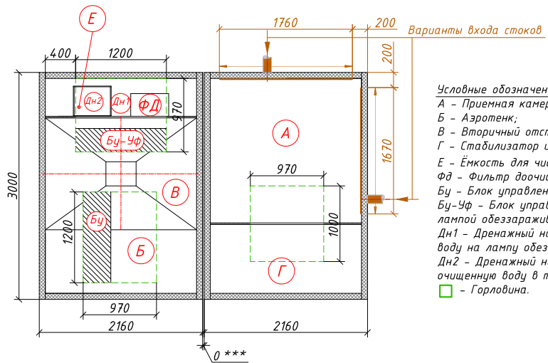
Схема станции
