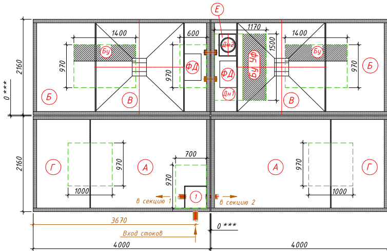
Схема станции
