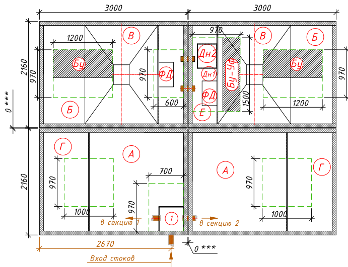
Схема станции
