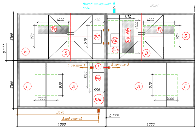
Схема станции
