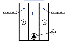
Схема распределения стоков КНС
