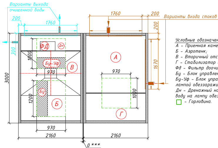
Схема станции
