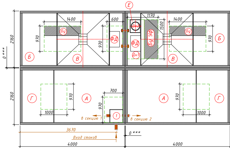
Схема станции
