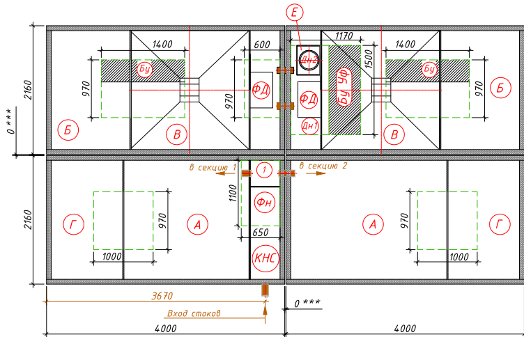
Схема станции
