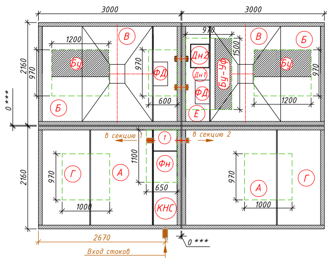
Схема станции
