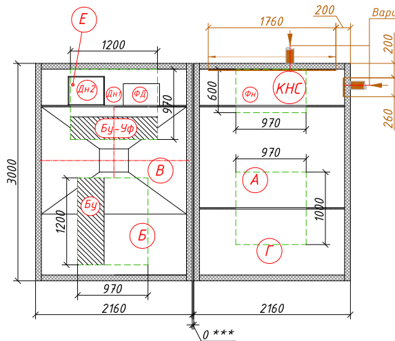
Схема станции
