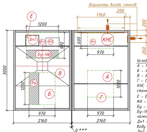
Схема станции
