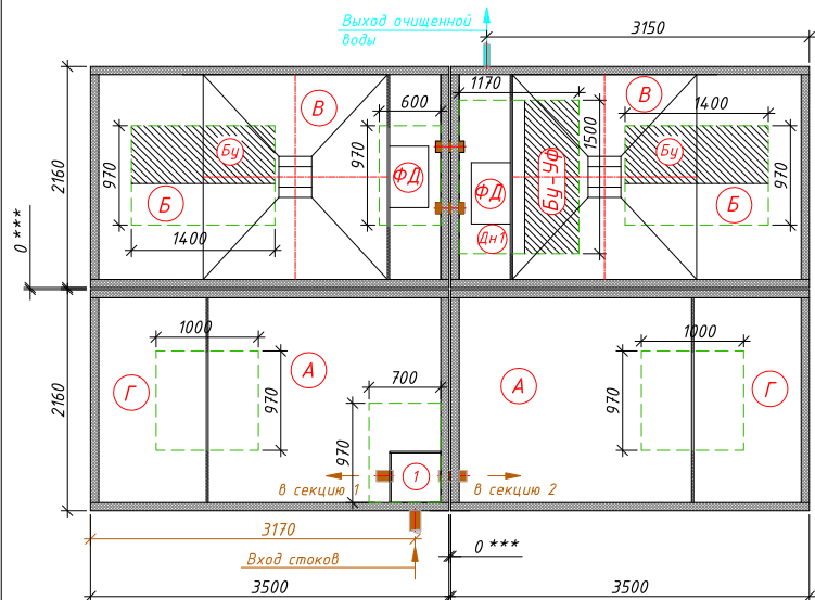
Схема станции
