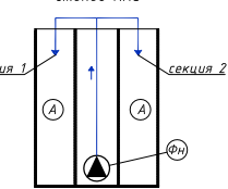
Схема распределения стоков КНС
